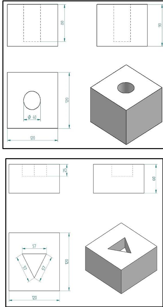
Şekil 5- Platformun Boyutları
