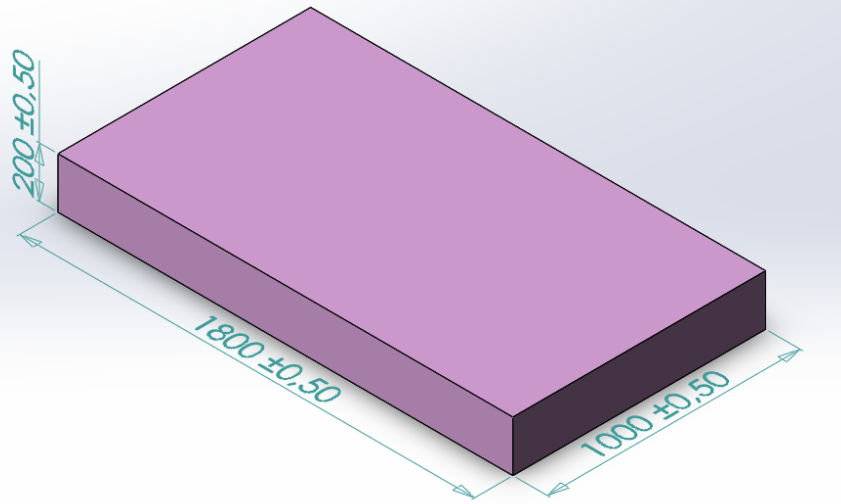
Şekil-18 İç Alana Girmek İçin Üzerinden Geçilecek Yükselti Platformunun Ölçüleri
