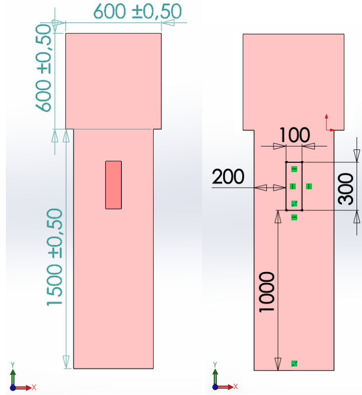
Şekil-20 Göbeklitepenin İçerisinde Bulunan T Sütunu Ölçüleri
