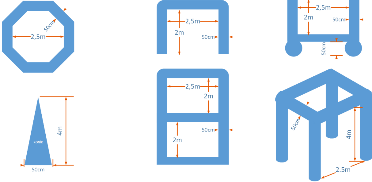
Şekil 23. Yarışma Alanındaki Parkurda Yer Alması Ön Görülen Engel Çeşitleri ve Ölçüleri.
